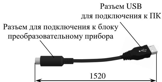
Рисунок 1.1 – Кабель связи с ПК КС303/603/903 ВР48.04.100
