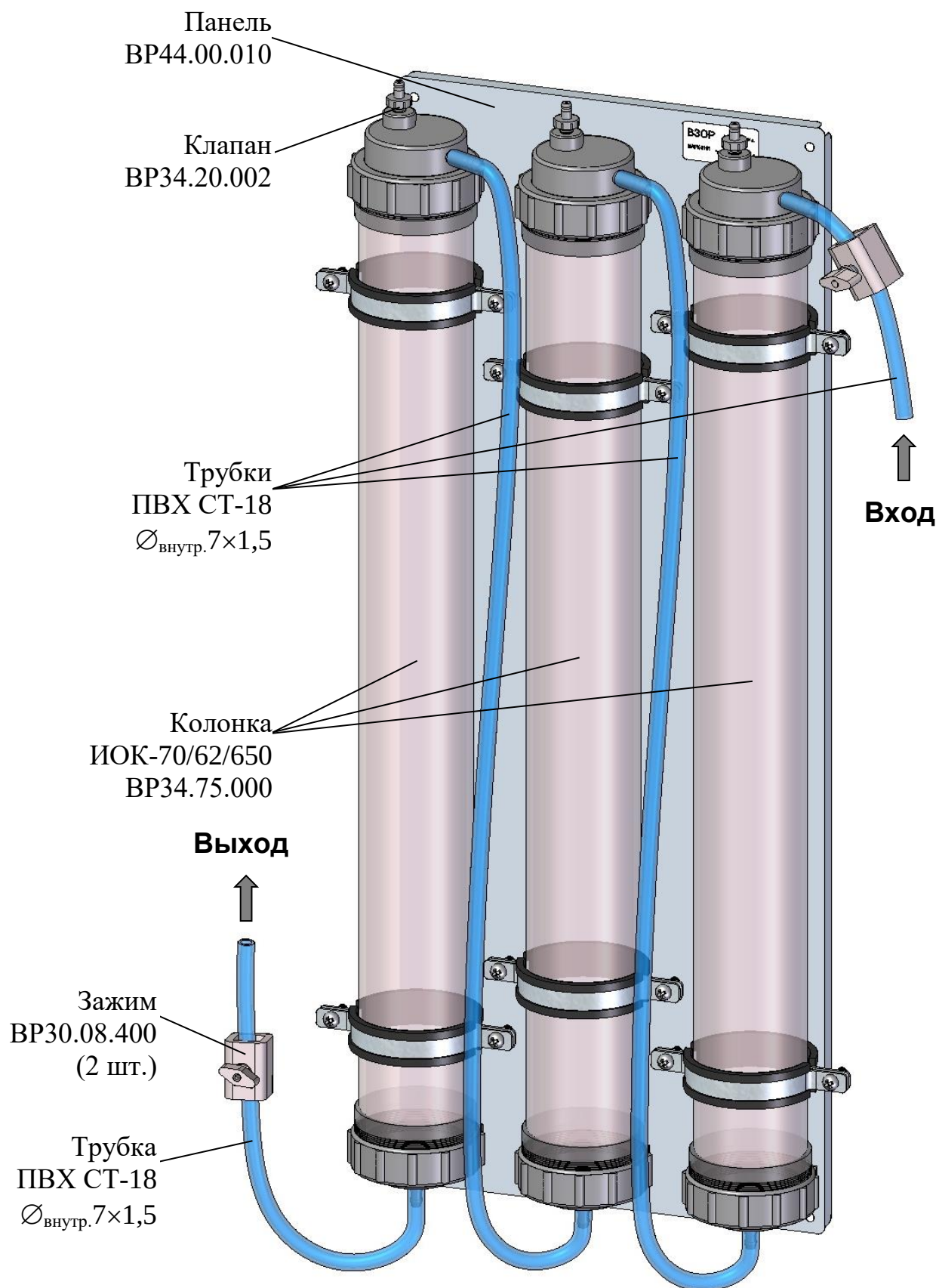
Рисунок 1.1 – Модуль MARK-3101
